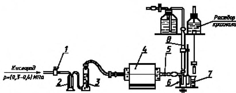
1 — кислородный баллон по ГОСТ 5583 с редукционным вентилем 2 — склянка Тищенко, содержащая раствор марганцово-кислого калия массовой концентрации 0,04 г/см 3 в растворе гидроксида калия массовой концентрации 0,4 г/см 3 ; 3 — сушильная колонка, заполненная хлористым кальцием 4 — трубчатая печь с карборундовыми нагревателями 5 — фарфоровая (высокоглиноземистая) трубка длиной 750—800 мм и внутренним диаметром 20—26 мм 6 — сосуд для титрования; 7 — сосуд для сравнения 8 — бюретка
