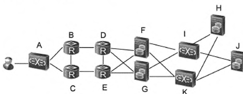
Рисунок A.1 — Пример типичной топологии сети E2E
