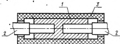
1 — стержень; 2 — кабель; 3 — корпус
