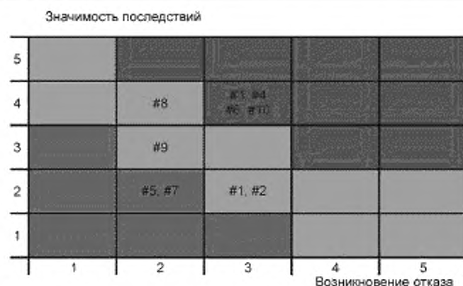
Рисунок С.3 — Матрица критичности для отчета FMECA в соответствии с таблицей С.5, разработанная в виде двумерного изображения, без учета обнаруживаемости
