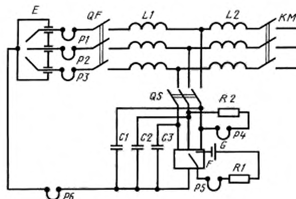
E — экспериментальная установка; QF — автоматический выключатель; QS — автоматический выключатель; L1, L2 — кабельные вставки; KM — магнитный пускатель; P1—P6 — резисторы; G — источник питания; R1, R2 и R3 — сопротивления; C1, C2, C3 — емкости; F — аппарат защиты
