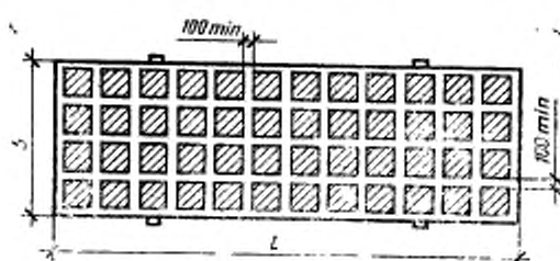
Расположение нагрузки на плите в плане
