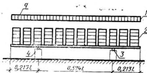
Схема опирания плиты
