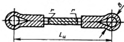
Машина для испытаний с кнехтами для наращенных петель (отметка r расположена на расстоянии 150 мм от последнего витка сращивания)
