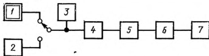
1 — передатчик (радиостанция в режиме передачи); 2 — высокочастотный генератор сигналов; 3 — высокочастотный вольтметр переменного тока; 4 — испытательная нагрузка; 5 — фиксированный attenuатор; 6 — режекторный фильтр; 7 — измерительный приемник
