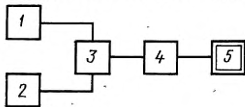
1, 2—высокочастотные генераторы сигналов; 3—согласующее устройство 1-го типа; 4—испытательная нагрузка; 5—радиостанция
