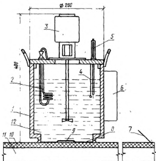
1 — сосуд цилиндрической формы; 2 — электронагреватель трубчатый; 3 — электрошпатель; 4, 7 — термодатчики; 5 — электроконтактный термометр; 6 — блок управления; 8 — дно из полиэтиленовой или поливинилхлоридной пленки; 9 — тепломер (измеритель теплового потока); 10 — испытуемый образец; 11 — бетонная плита; 12 — дистиллированная вода
