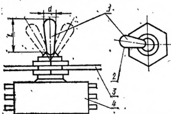
1 — приводной элемент; 2 — рабочая поверхность; 3 — панель; 4 — тумблер Черт. 1
