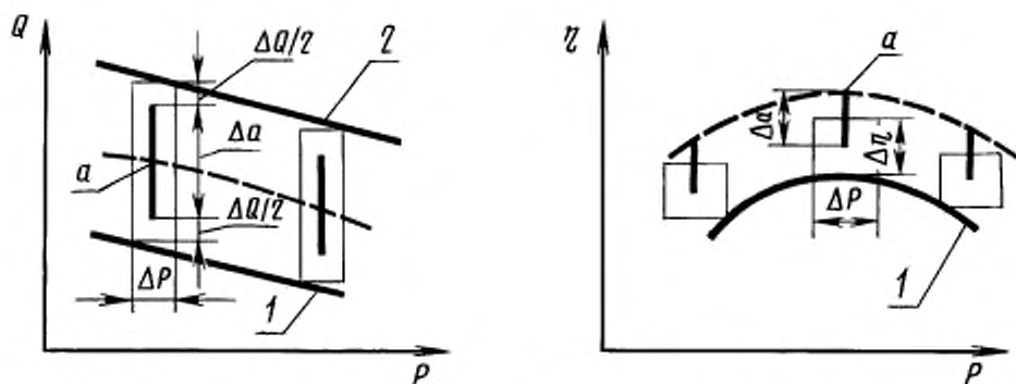
1 и 2 — кривые, ограничивающие полосу допустимых отклонений; a — номинальное значение параметра; \Delta a — допуск на параметр; \Delta P , \Delta Q , \Delta a — относительные погрешности результатов испытаний
