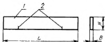
1 — рабочая поверхность; 2 — риски, отмечающие точки наименьшего прогиба
