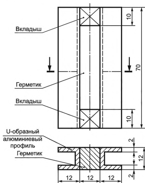
Рисунок Д.1 — Образец шва для испытаний
