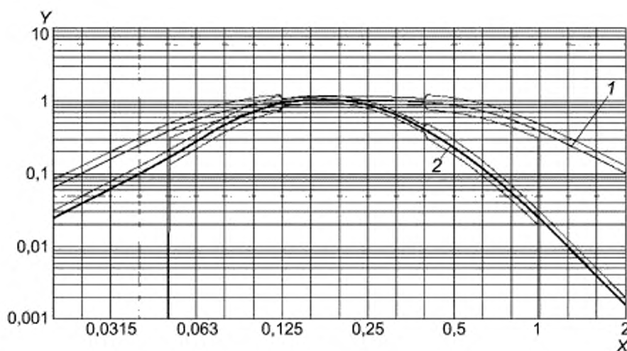
Рисунок В.9 — Модуль функции частотной коррекции W_f
