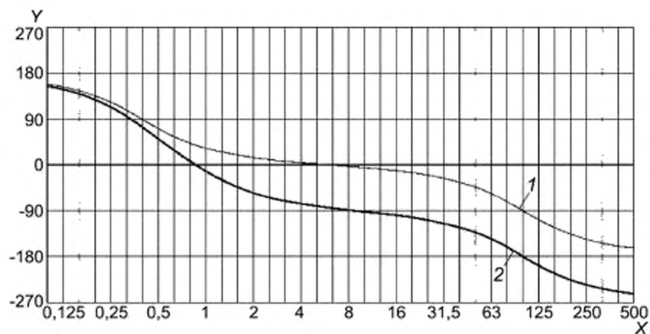
Рисунок В.8 — Фаза функции частотной коррекции W_e
