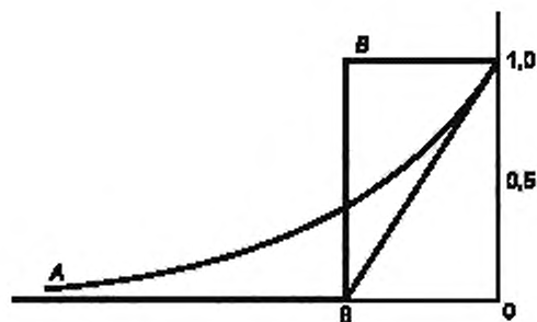
А — экспоненциальное окно; В — прямоугольное окно линейного интегрирования
