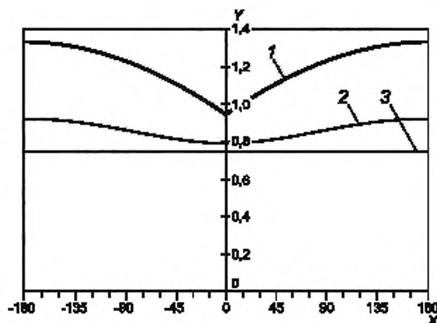
X — фазовый сдвиг гармоник, ...°; Y — значение параметра вибрации; 1 — пиковое значение \text{м/с}^2 ; 2 — доза вибрации, \text{м/с}^{-1.75} ; 3 — с.к.з., \text{м/с}^2
