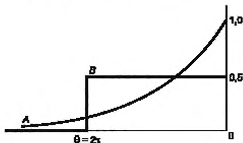
А — экспоненциальное окно; В — прямоугольное окно линейного интегрирования; \theta — период линейного интегрирования; \tau — постоянная времени экспоненциального усреднения
