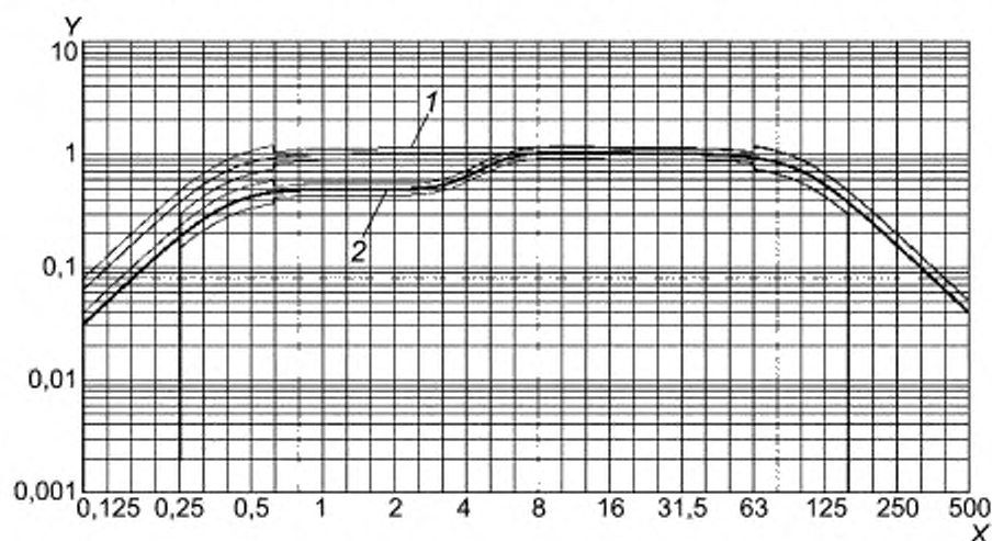
Рисунок В.13 — Модуль функции частотной коррекции W_f
