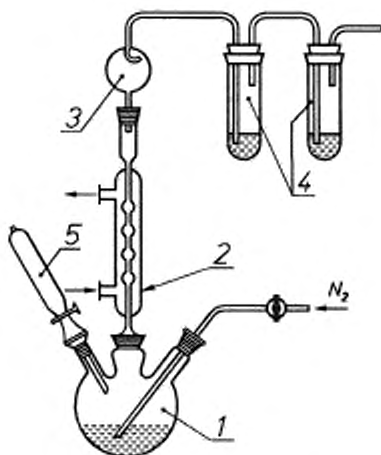
1 — трехгорлая колба; 2 — холодильник; 3 — каплеуловитель; 4 — приемные пробирки (барботеры); 5 — капельная воронка
