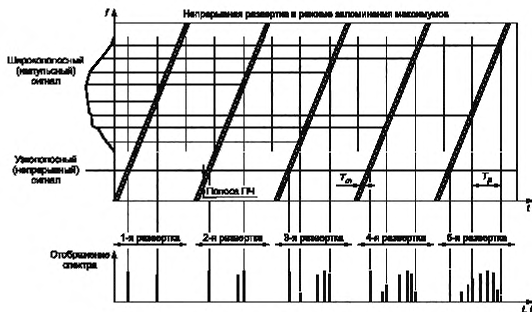
T_{из} — время измерения; T_{п} — период повторения импульсов широкополосных ИРП. Моменты появления импульсов показаны вертикальными линиями на верхней части рисунка.
