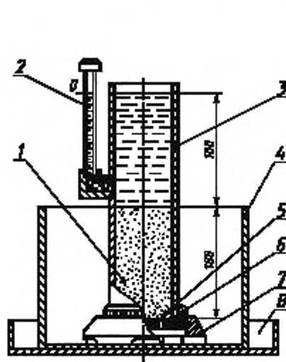
1 — образец; 2 — пьезометр; 3 — трубка; 4 — стакан; 5 — сетка; 6 — перфорированное съемное дно; 7 — подставка; 8 — поддон
