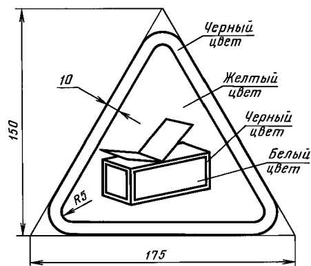
Черт. 1
