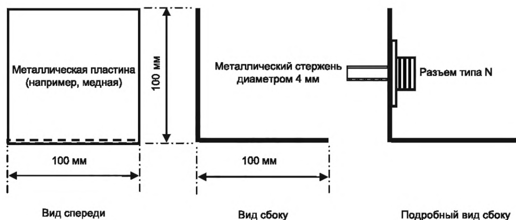
Рисунок A.3 — Размеры опорной пластины
