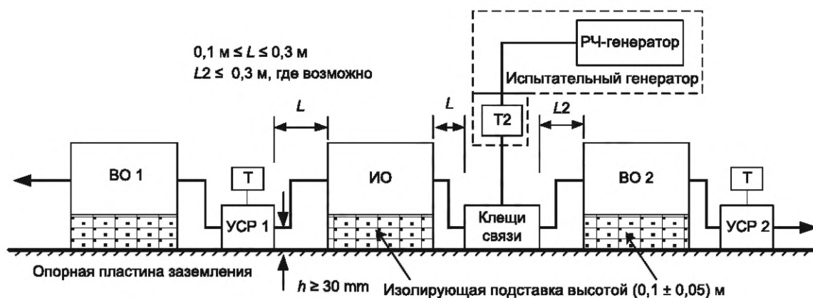
Схема расположения оборудования, используемого для клемм связи при испытаниях на устойчивость к помехам
