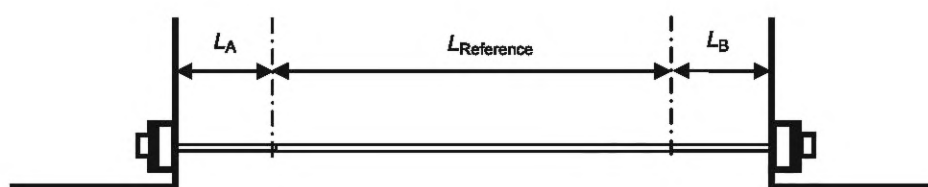
Рисунок A.4 — Испытательное приспособление
