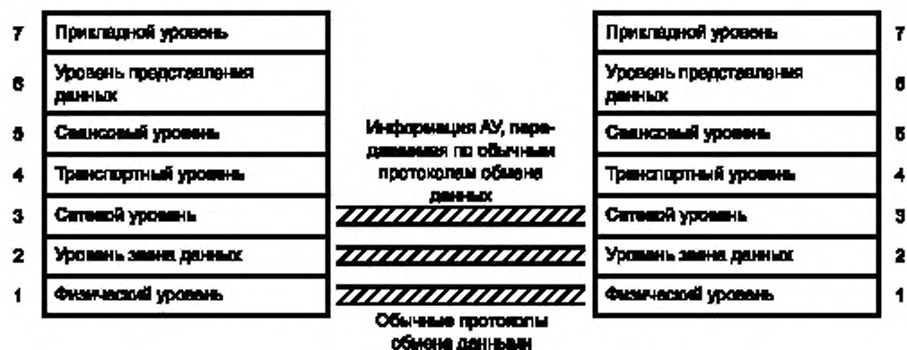
Рисунок А.3 — Операции (N)-уровня
