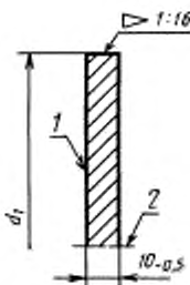
Калибр-пробка типа Г-У
