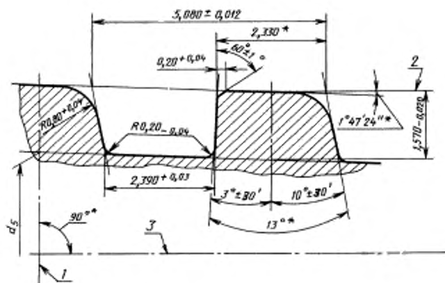
Профиль резьбы калибра-пробки типа Р
