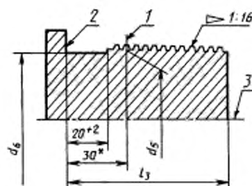
Калибр-пробка типа Р
