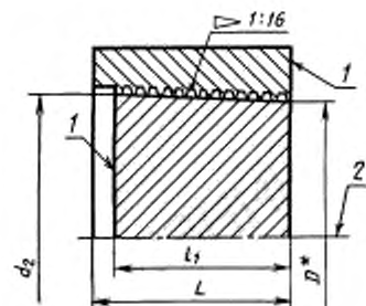
Калибр-кольцо типа Р и калибр-пробка типа К-Г-Р
