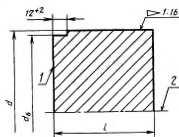
Калибр-пробка типа Г
