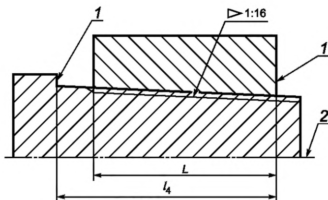
Рисунок 8 — Калибр-кольцо типа Г-У и калибр-пробка типа К-Г-Г-У
