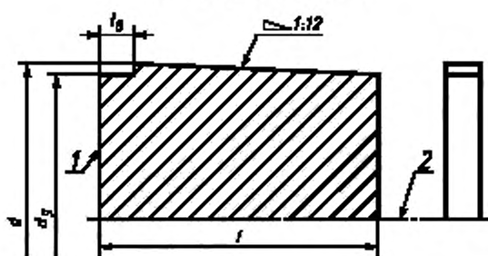
Калибр-пробка типа Г-Н
