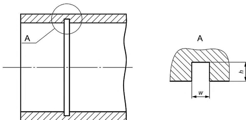
Рисунок Б.7 — Настроечный образец с кольцевым плоскодонным пазом при настройке чувствительности для выявления расслоений
