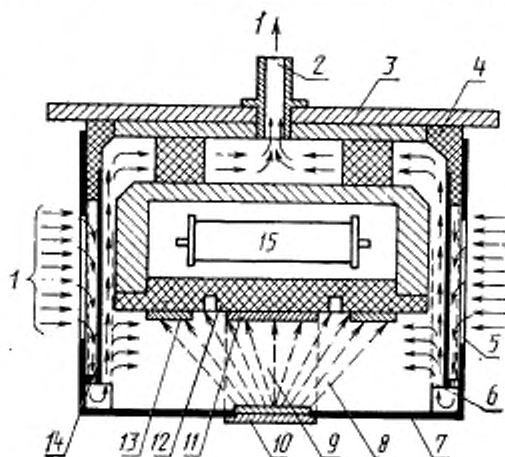
Принцип действия контрольной ионизационной камеры (КИК)
