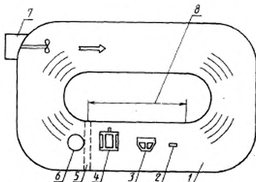
Испытательная камера
