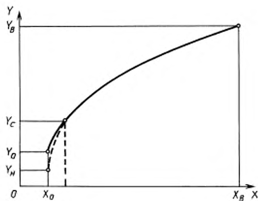
Черт. 2. Нелинейная зависимость y - y_n = a\sqrt{x - x_0}
