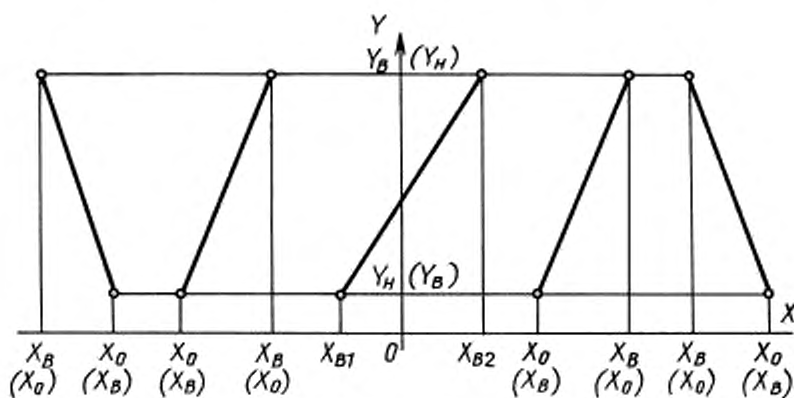
Черт. 1. Линейная зависимость y - y_n = k(x - x_0) ; x_a , x_{a1} , x_{a2} — верхние пределы измерений; для линейно убывающей характеристики значениям (x_0) и (x_a) соответствуют значения выходного сигнала (y_n) и (y_a)
