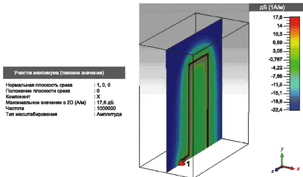
Рисунок Е.9 — Двумерный график магнитного поля H_x в плоскости y — z для стандартной индукционной катушки размером 1 м × 2,6 м
