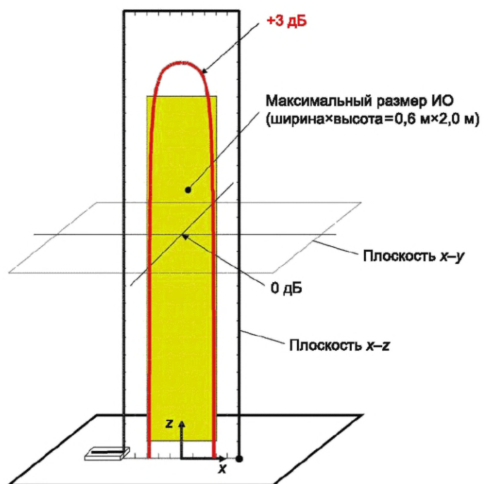
Рисунок А.4 — Изолиния +3 дБ напряженности магнитного поля (предельные значения) в плоскости x-z для индукционной катушки размером 1\text{ м} \times 2,6\text{ м} с опорной пластиной заземления
