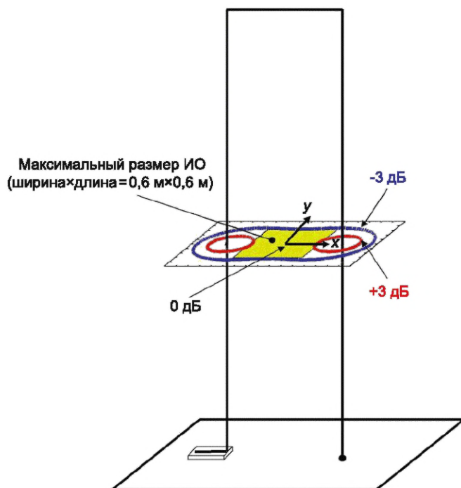
Рисунок А.5 — Изолинии +3 дБ и -3 дБ напряженности магнитного поля (предельные значения) в плоскости x-y для индукционной катушки размером 1\text{ м} \times 2,6\text{ м} с опорной пластиной заземления
