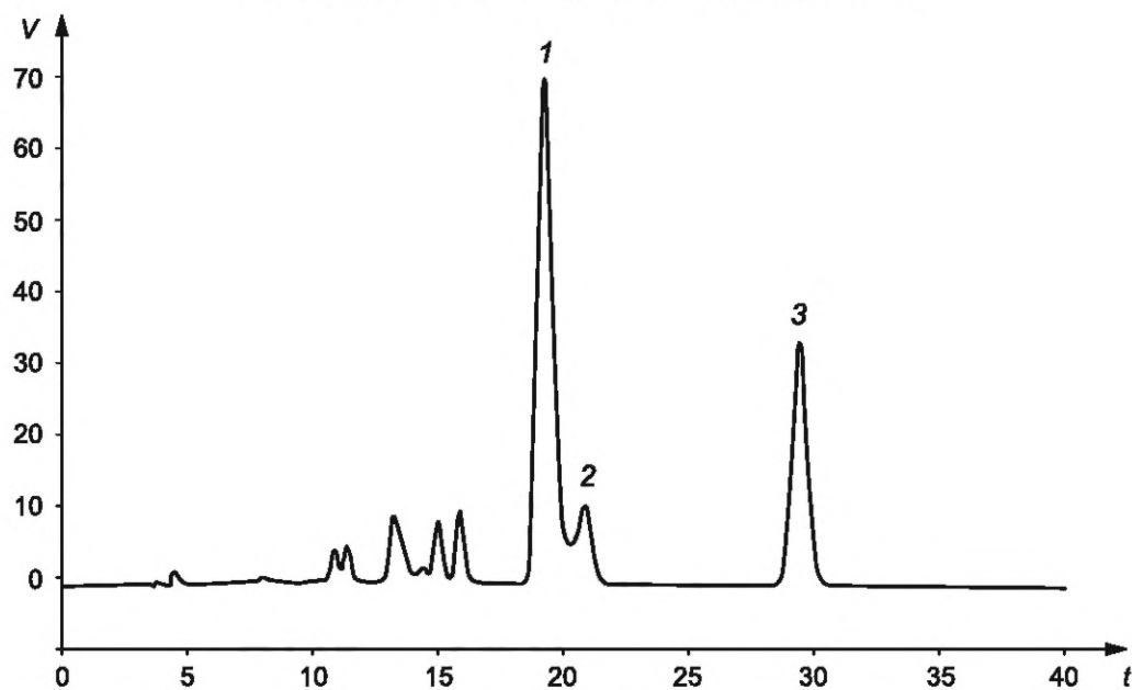
Рисунок А.1 — Хроматограмма ВЭЖХ оливкового масла первого холодного отжима с массовой долей пиррофеофитина 5 % в продуктах распада хлорофилла
