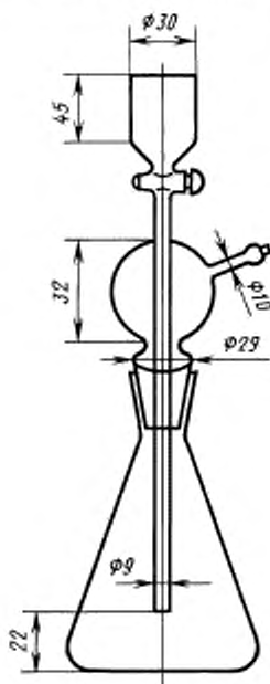
Прибор для растворения металлического олова
