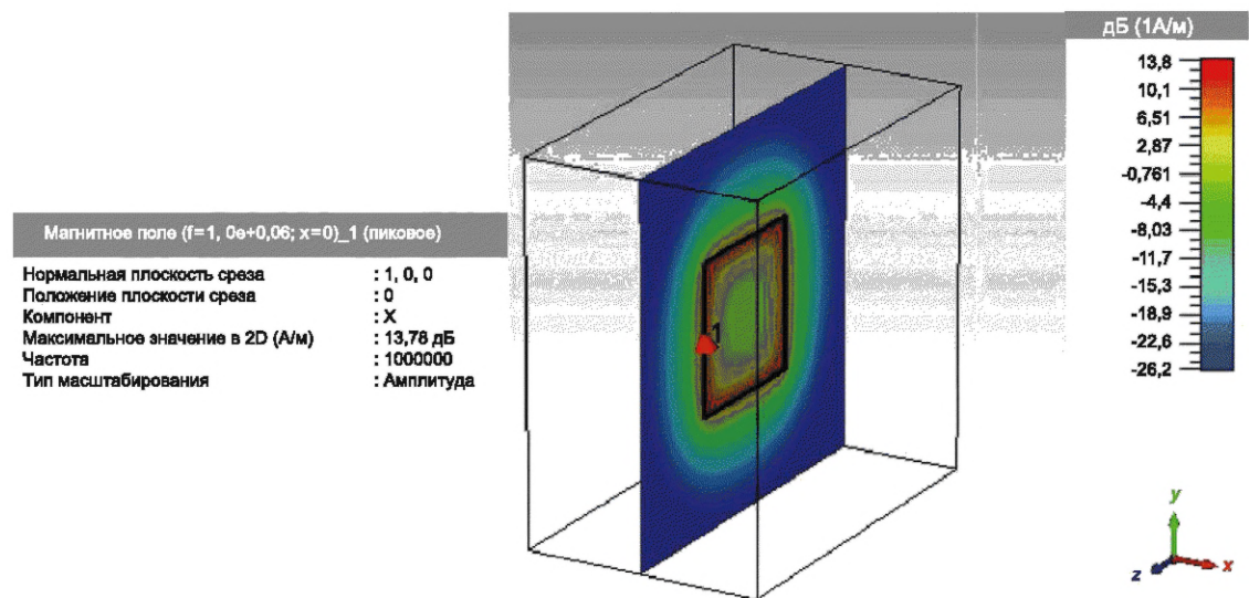
Рисунок G.6 — График магнитного поля H_x в плоскости y-z для индукционной катушки размером 1 × 1 м
