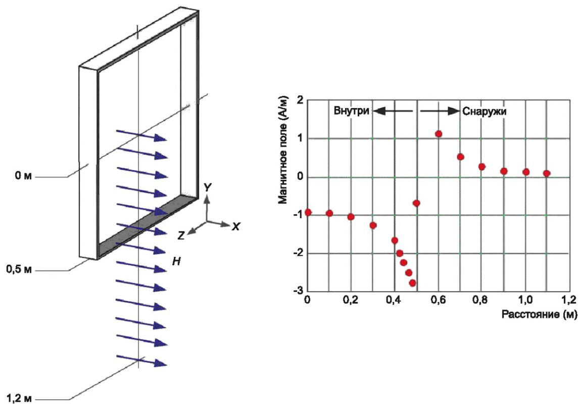
Рисунок G.2 — Значение магнитного поля H_x , А/м, вдоль стороны индукционной катушки размером 1 \times 1 м
