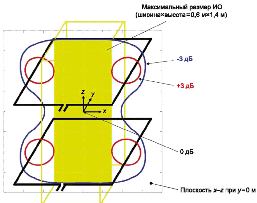
Рисунок F.3 — Изолинии +3 дБ и -3 дБ напряженности магнитного поля (предельные значения) в плоскости x - z для системы, состоящей из двойной индукционной катушки, расстояние между которыми составляет 0,8 м
