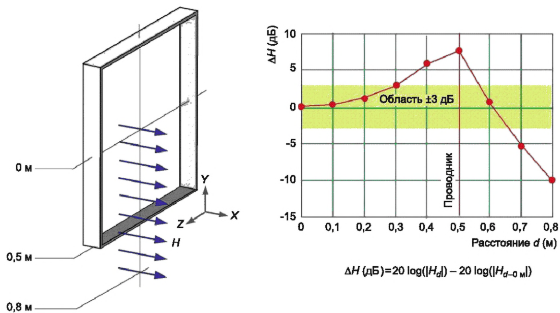
Рисунок G.4 — Значение магнитного поля H_x , дБ, вдоль стороны для индукционной катушки размером 1 \times 1 м
