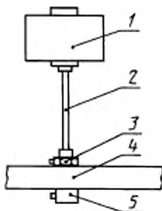
1 — вибровозбудитель; 2 — толкатель; 3 — преобразователь силы; 4 — испытываемая конструкция; 5 — акселерометр
