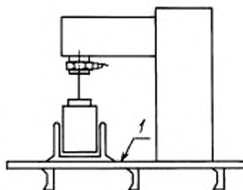
в) Пример неправильной установки вибровозбудителя
