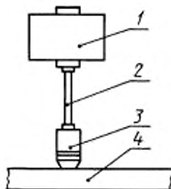
1 — виброизбудитель, 2 — толкатель, 3 — импедансная головка 4 — испытываемая конструкция
