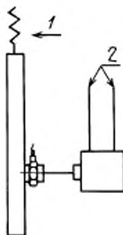
б) Реакция инерции вибровозбудителя
