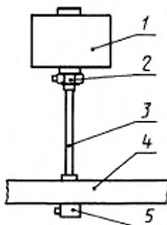
1 — виброисполнитель, 2 — преобразователь силы, 3 — толкатель; 4 — испытываемая конструкция; 5 — акселерометр
