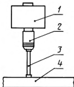
1 — виброисполнитель, 2 — импедансная головка; 3 — толкатель; 4 — испытываемая конструкция
