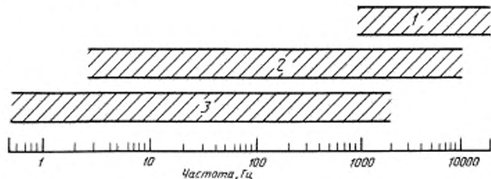
1 — пьезоэлектрические вибровозбудители; 2 — электродинамические вибровозбудители; 3 — электрогидравлические вибровозбудители
