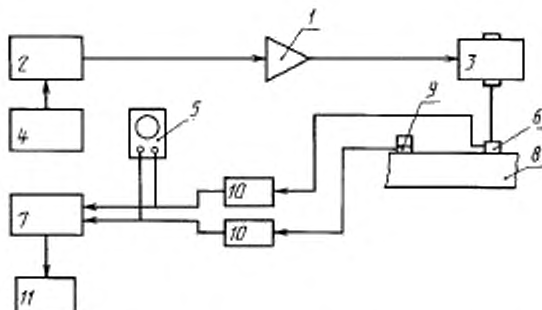
1 — усилитель мощности, 2 — устройство регулировки амплитуды, 3 — вибровозбудитель, 4 — генератор сигналов, 5 — контрольный осциллограф, 6 — преобразователь сил, 7 — анализатор, 8 — испытуемая конструкция, 9 — преобразователь вибрации, 10 — формовщик сигнала, 11 — графоинструмент для другой выходной прибор
