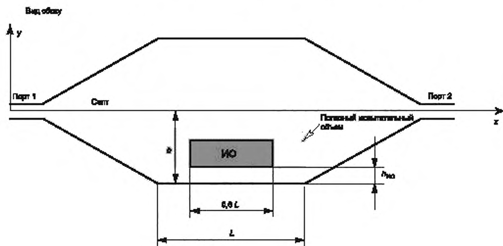
Рисунок А.6а — Вид сбоку
