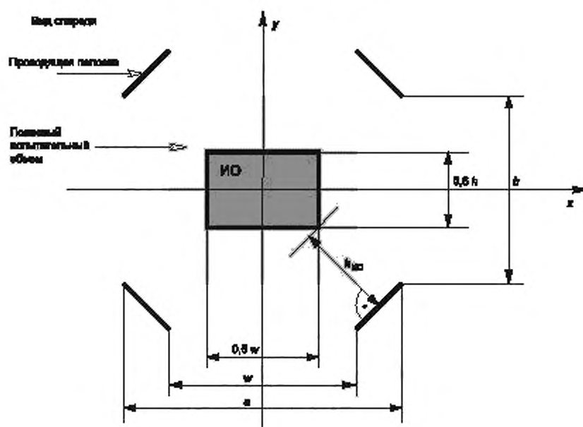
Рисунок A.9b — Поперечное сечение волновода
