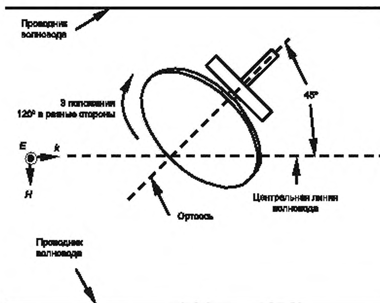
Рисунок A.2c — Вид сверху (пояснение пунктов 3.1.21 и A.5.2)
