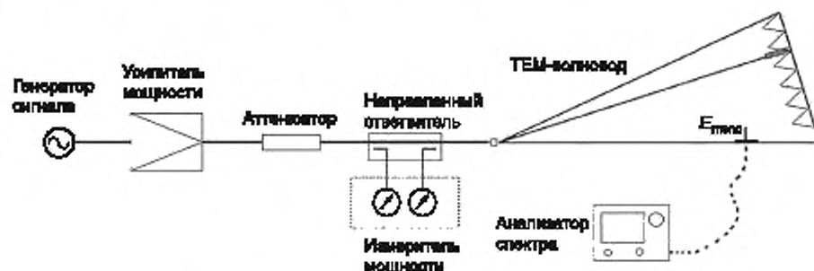
Рисунок E.5.a — Применение монополярной антенны
