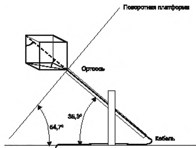
Рисунок A.2b — Вид сбоку (пояснение пунктов 3.1.21 и A.5.2)
