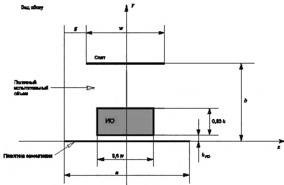
Рисунок А.8с — Поперечное сечение волновода
