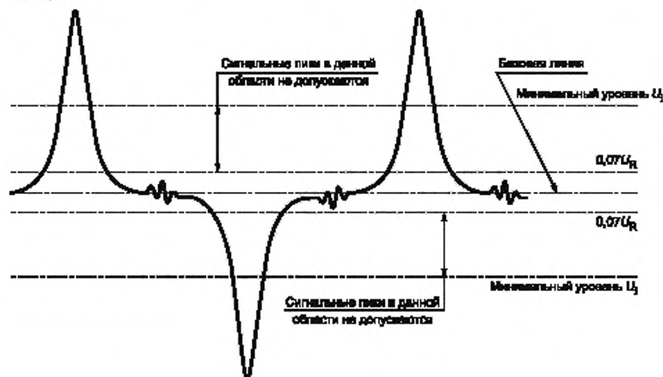
Рисунок 9 — Присутствие нежелательных пиков в форме сигнала
