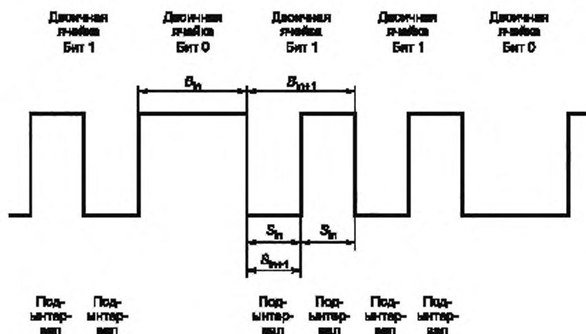
Рисунок 10 — Изменение промежутка между переходами потока
