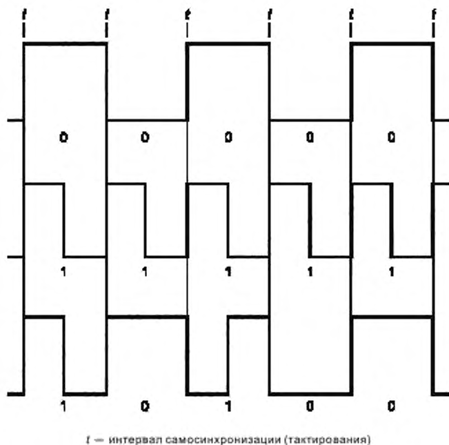
Рисунок 7 — Пример двухчастотного синфазного кодирования
