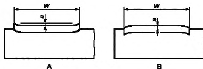
Рисунок 3 — Профиль поверхности
