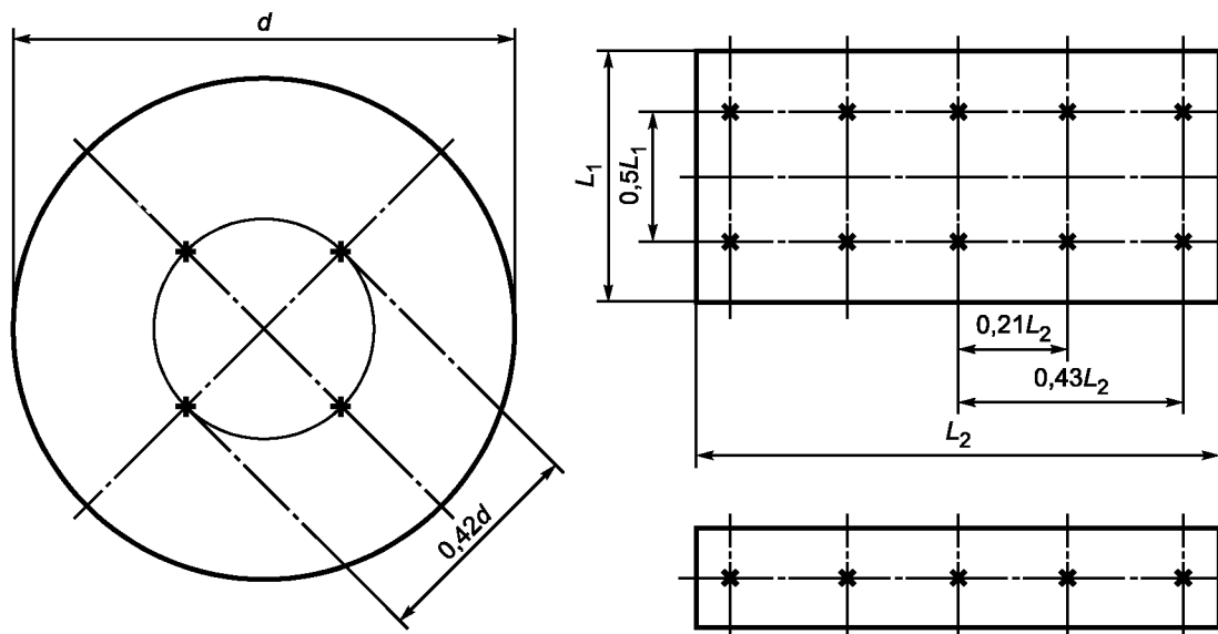
Рисунок 1 — Установка температурных датчиков
