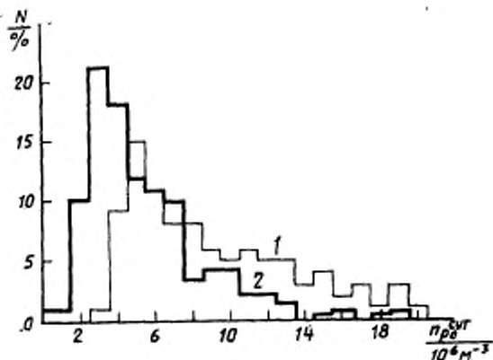
1—распределение в минимуме 11-летнего цикла; 2—распределение в максимуме 11-летнего цикла; N —частота попадания результатов измерения n_{p_0}^{\text{сут}} в интервал
