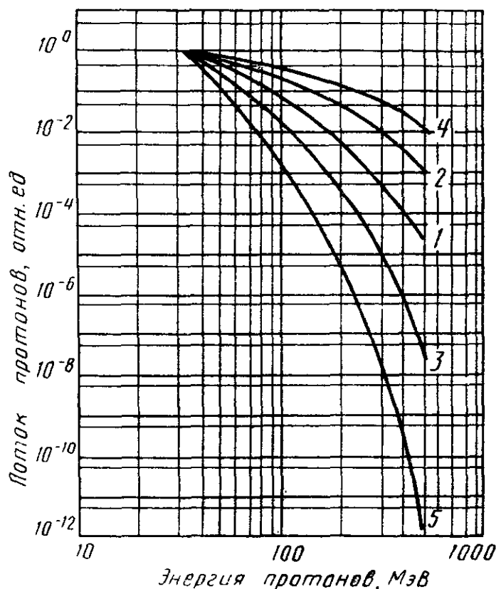
Интегральные энергетические спектры для различных R_0
