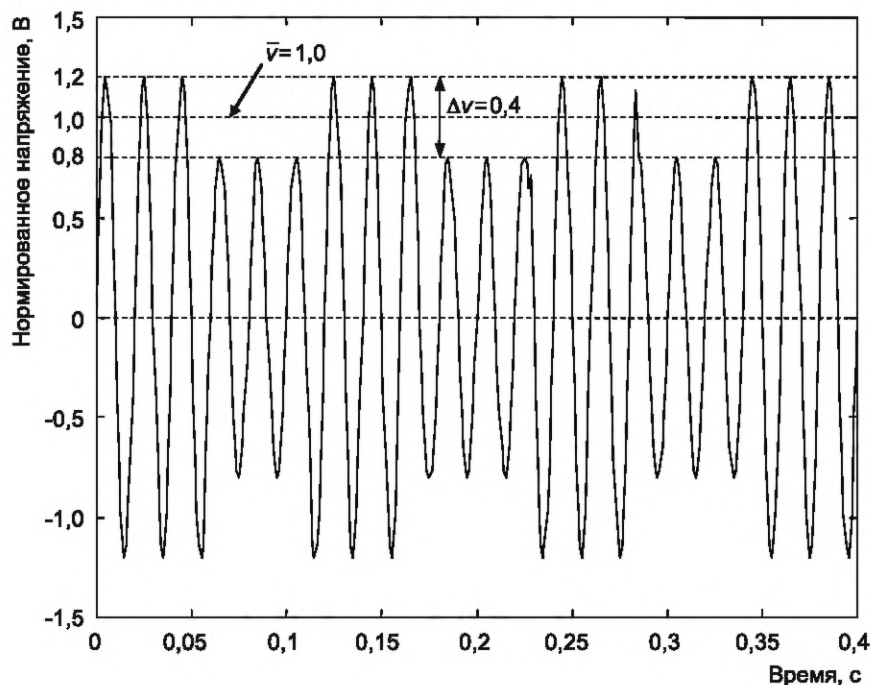
Рисунок В.1 — Прямоугольное изменение напряжения \Delta U/U = 40 %, 8,8 Гц, 17,6 изменений/в секунду
