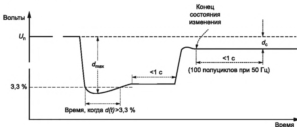
Рисунок В.2а — Пример определения параметра «d»
