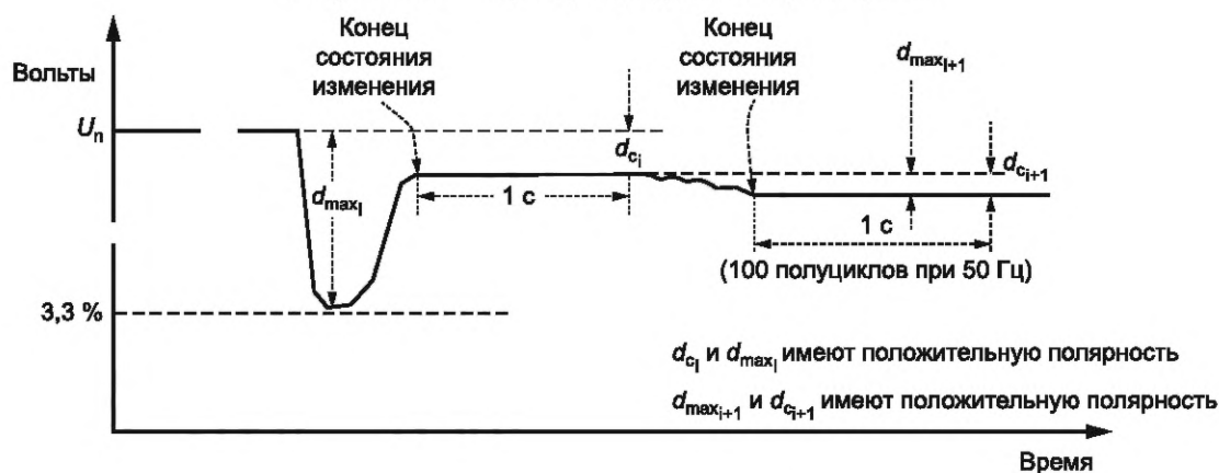
Рисунок В.2а — Пример определения параметра «d»
