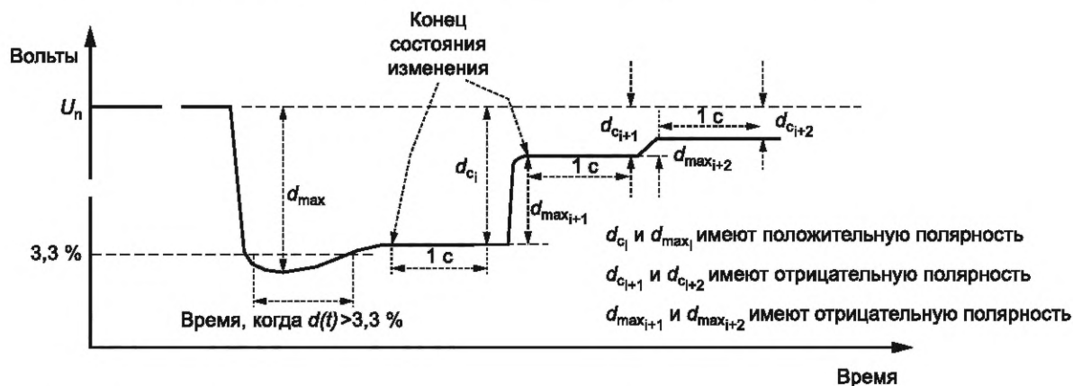
Рисунок В.2с — Пример определения множественного устойчивого состояния и последовательности и полярности d_{max} и d_c
