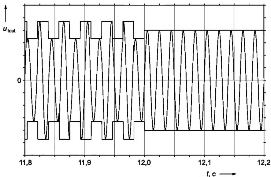
Рисунок 1 — Испытательное напряжение, модулированное прямоугольным сигналом частотой 28 Гц с 20-процентным рабочим циклом
