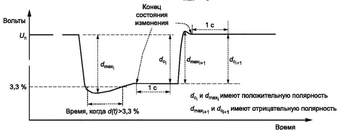
Рисунок В.2д — Пример определения последовательности и полярности d_{max} и d_c при многократных установившихся состояниях
