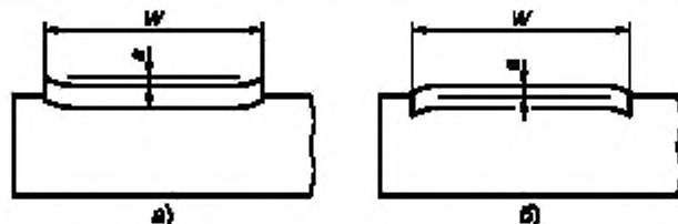
Рисунок 3 — Профиль поверхности
