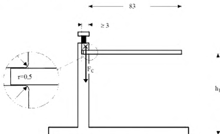
Рисунок А.1 — Карта в зажимном устройстве до воздействия температуры
