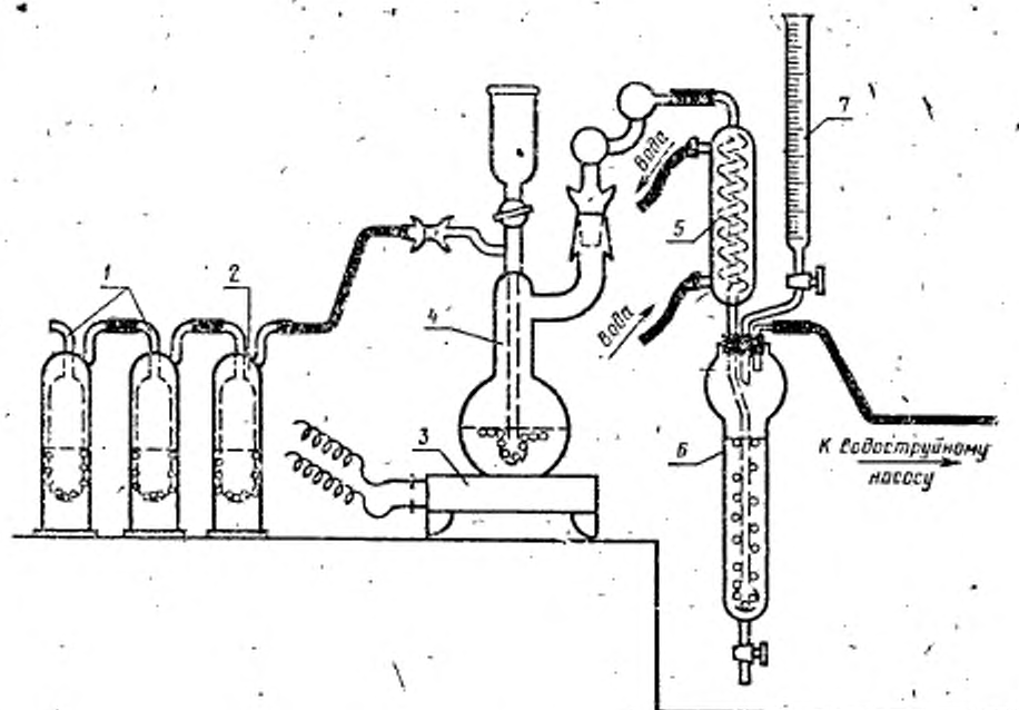
1—склянки-ловушки, заполненные серной кислотой; 2—склянка-ловушка, заподненная водой; 3—электроплитка; 4—дистилляционная колба из термостойкого стекла вместимостью 500 мл с припаянной пробкой, снабженной капельной воронкой с краном; 5—холодильник; 6—сосуд для улавливания аммиака; 7—микробюретка 2-го класса
