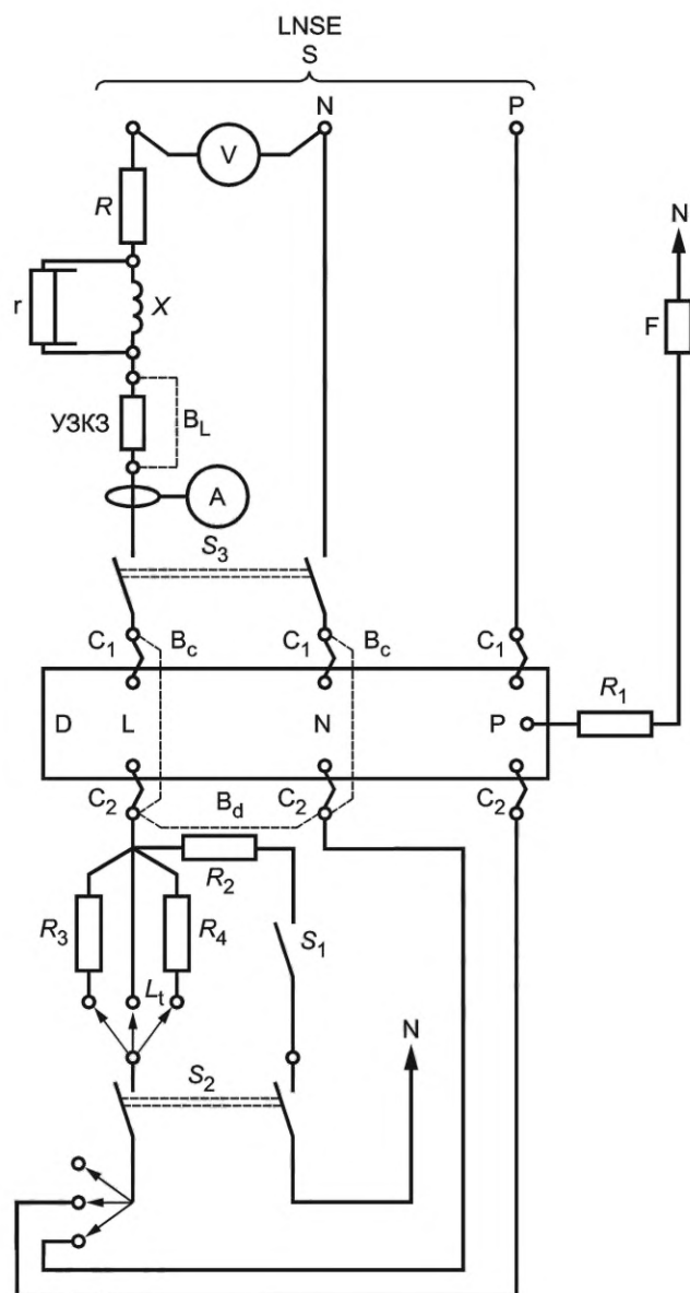
а) Тип LNSE/LNE
