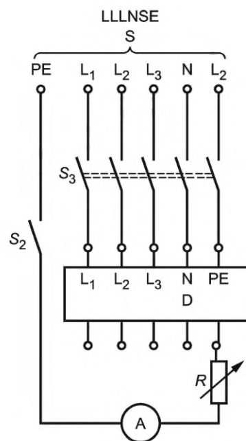
ф) Тип LLLNSE
