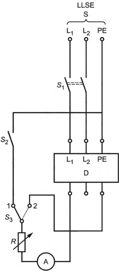
a) Тип LLSE/LLE
