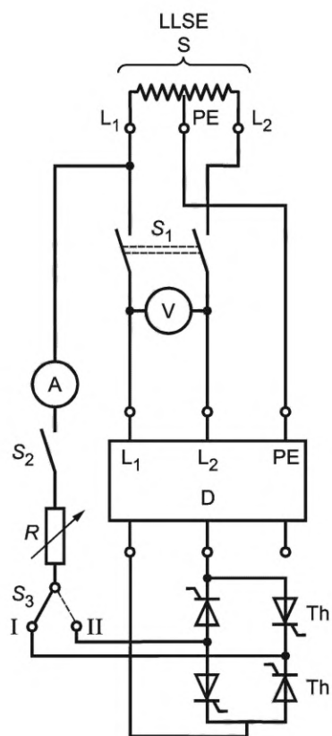
b) Типы LLSE/LLLE
