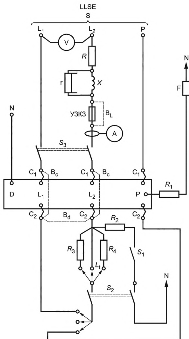
b) Тип LLSE/LE
