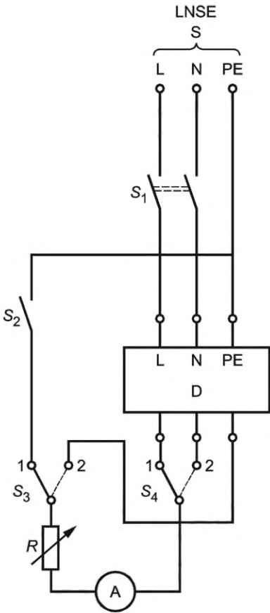
b) Тип LNSE/LNE
