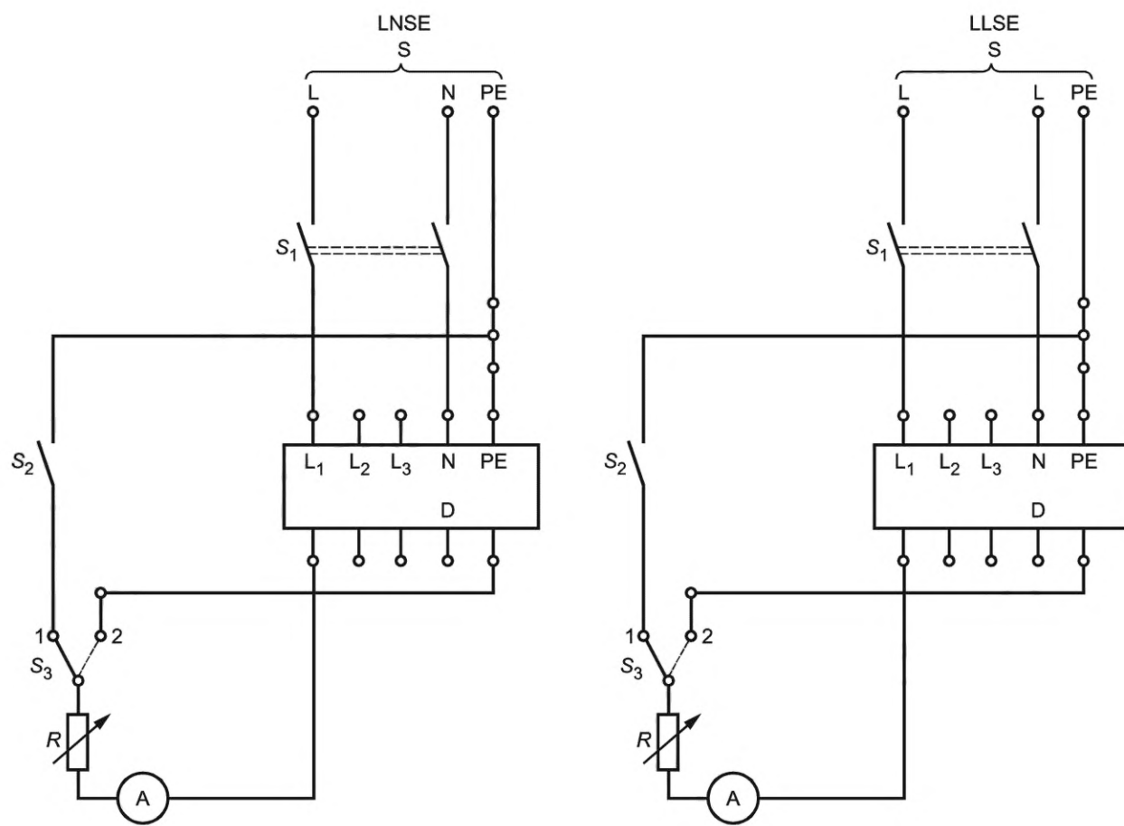
с) Тип LLLNSE/LLLNE в сети LNSE
