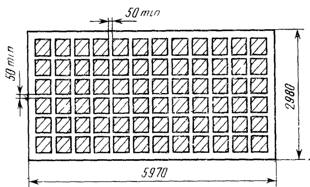
Расположение нагрузки на плите в плане
