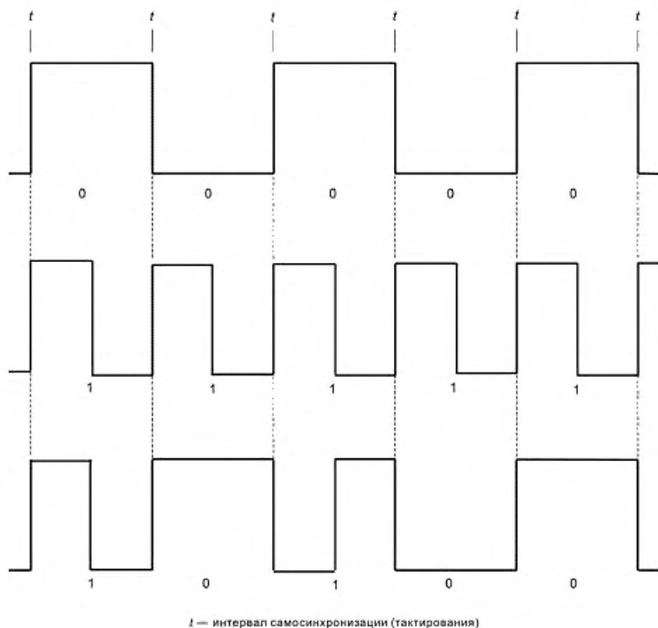
Рисунок 8 — Примеры двухчастотного синфазного кодирования
