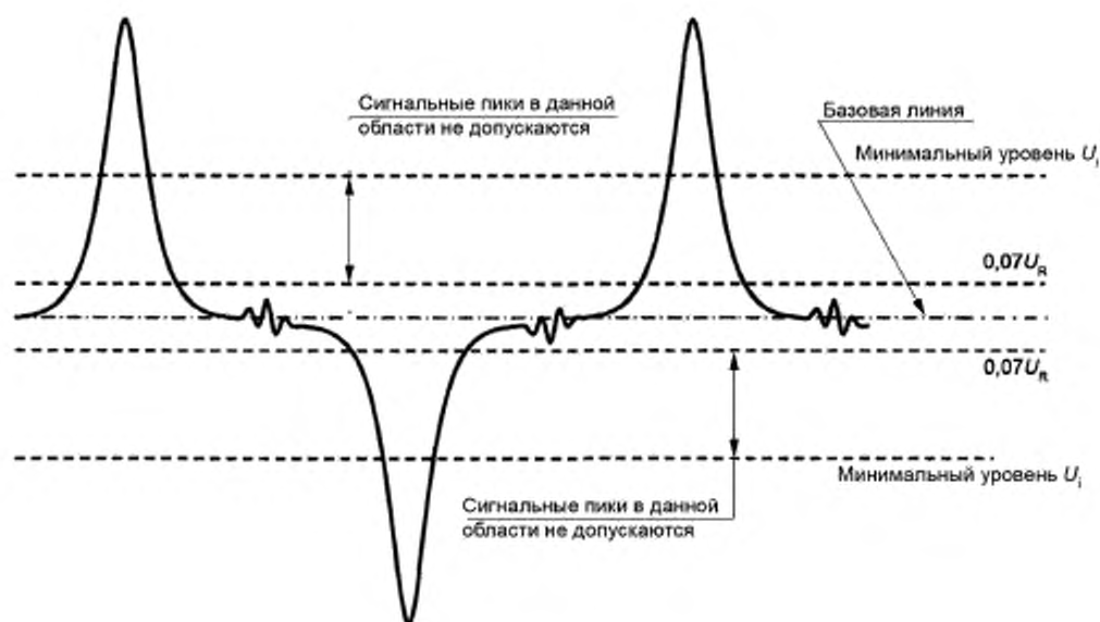
Рисунок 10 — Присутствие нежелательных пиков в форме сигнала
