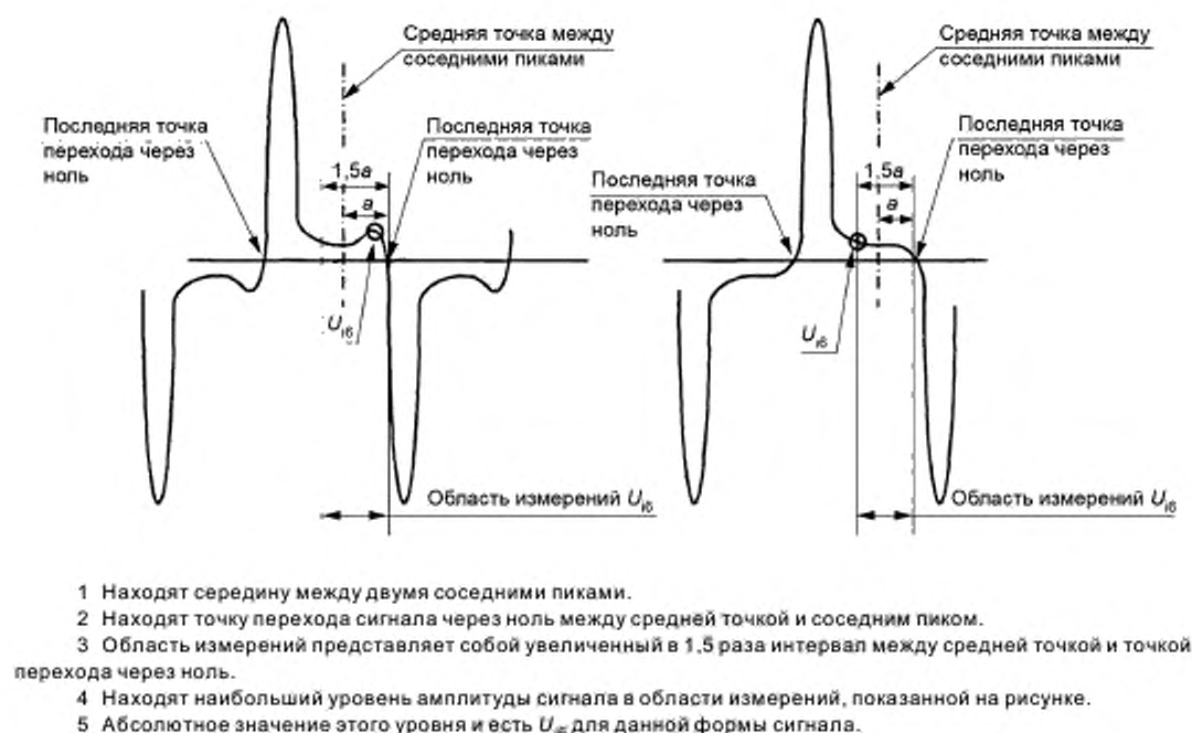
Рисунок 7 — Измерения формы сигнала
