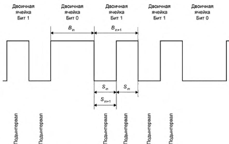
Рисунок 11 — Изменение промежутка между переходами потока
