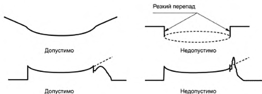
Рисунок 4 — Примеры профилей поверхности
