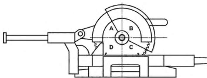
а) Торцовочная пила в крайнем нижнем положении
