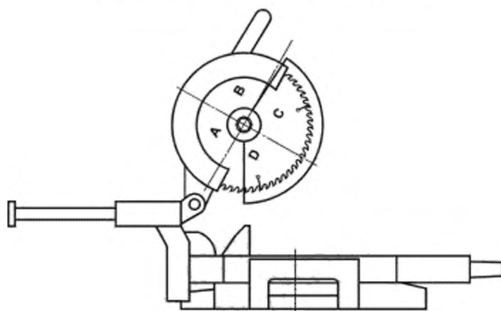
б) Торцовочная пила в крайнем верхнем положении
