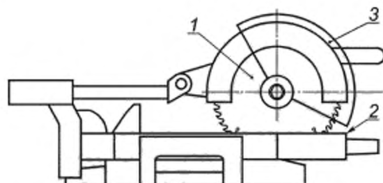
1 — пильный диск; 2 — конец стола; 3 — нижний защитный кожух
