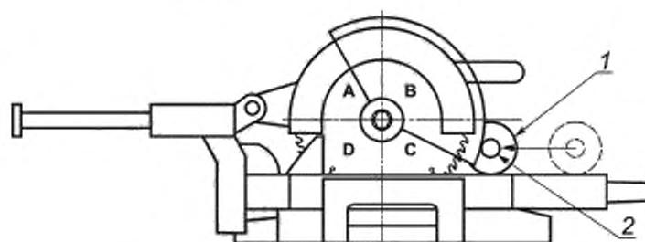
1 — фланец щупа; 2 — испытательный участок щупа
