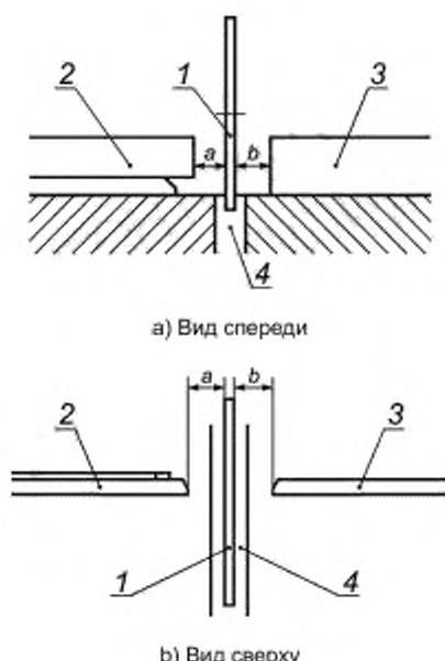
а, б — зазор между упором и стальным диском; 1 — стальной диск; 2 — регулируемая часть упора; 3 — нерегулируемый упор; 4 — паз в столе/вставке стола
