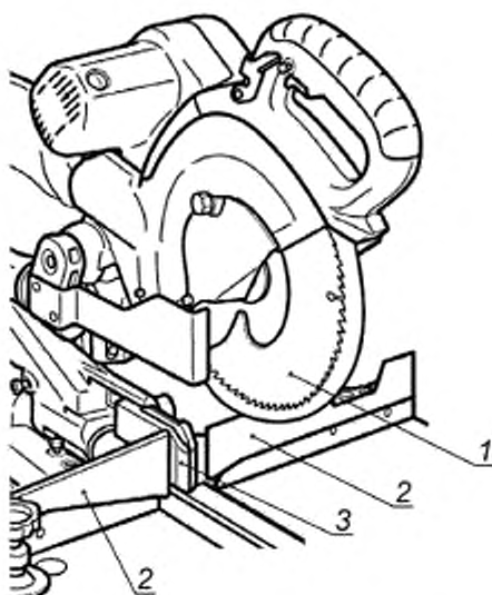
1 — пильный диск; 2 — упор; 3 — центральная поддержка объекта обработки
