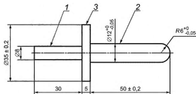
1 — участок рукоятки; 2 — испытательный участок; 3 — фланец щупа
