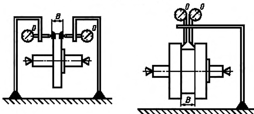
Схема измерения ширины фрез
