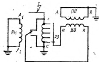
ПО — последовательная обмотка; ВО — обмотка возбуждения; РО — регулировочная обмотка
