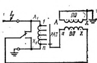
РАТ — регулировочный автотрансформатор
