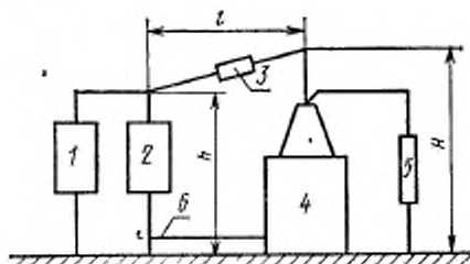
1 — генератор импульсных напряжений; 2 — срезающий разрядник; 3 — демпфирующее сопротивление; 4 — испытываемый объект; 5 — измерительное устройство (делитель напряжения); 6 — провод, соединяющий заземленный бак с заземленным срезающим разрядником
