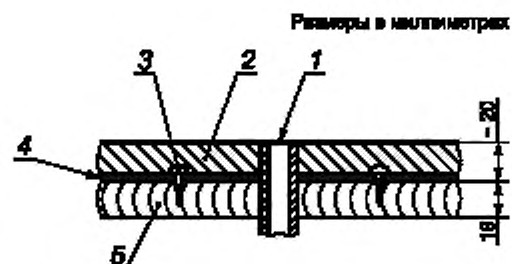
1 — верхняя часть трубки выброса находится на уровне или ниже поверхности покрытия; 2 — кокосовый коврик, 3 — гвоздь; 4 — основа из поливинилхлорида, 5 — основа из фанеры
