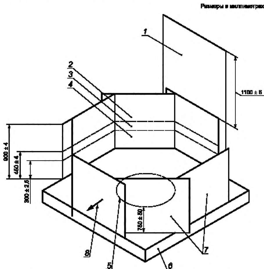
1 — верхняя зона — цель оператора (панель — цель из крафт-бумаги толщиной в один лист); 2 — верхняя зона-цель; 3 — средняя зона-цель; 4 — нижняя зона-цель; 5 — траектория лезвия; 6 — основание (см. рисунки ВВ.2 и ВВ.3); 7 — восемь панелей-целей из гофрированного картона с канавками по вертикали (см. рисунок ВВ.1); 8 — направление машины вперед
