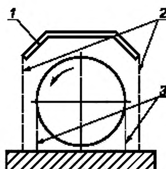
1 — защитный кожух; 2 — вертикальная проекция защитного кожуха; 3 — вертикальная проекция режущего устройства
