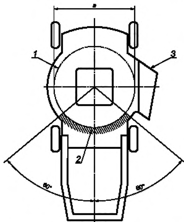
1 — траектория лезвия; 2 — область для исследования; 3 — разгрузочный желоб; a — ширина резания
