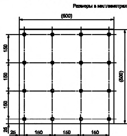
Рисунок ВВ.3 — Пример основания (вид сверху)
