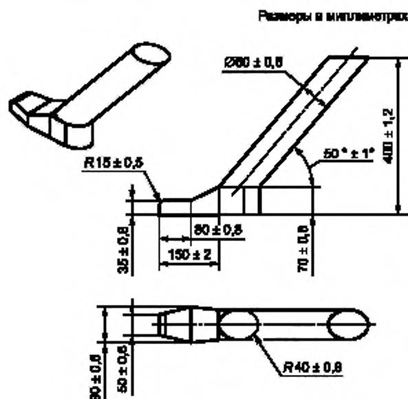
Рисунок СС.1 — Щуп в форме ноги
