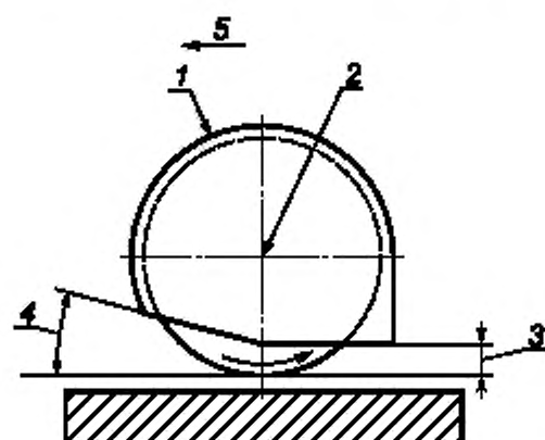
1 — минимальный защитный контур; 2 — ось вращения режущего устройства; 3 — высота защитного кожуха, сзади от оси вращения ( \leq 25 мм); 4 — угол наклона защитного кожуха вперед от оси вращения ( \leq 15^\circ ); 5 — направление движения
