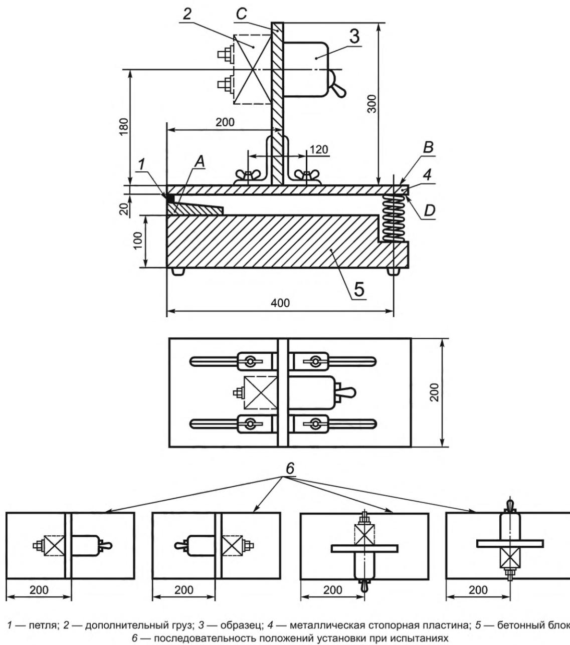
Рисунок 11 — Испытательная установка для испытания механическим воздействием (9.12.1)
