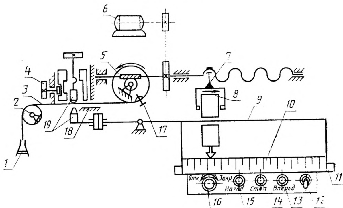
Схема прибора РТ-2М
