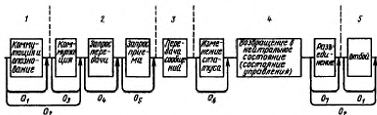
Диаграмма следования фаз
